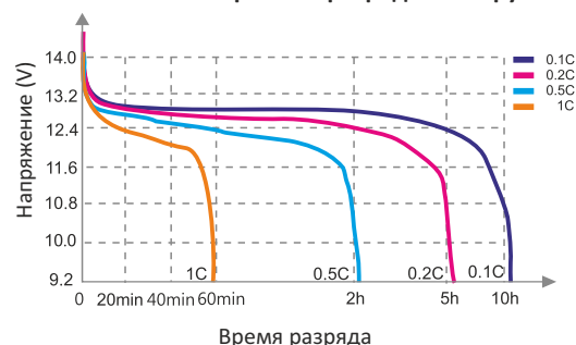
Зависимость времени разряда от нагрузки
