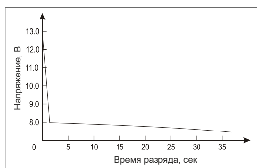
Разрядные характеристики (-18°С)
