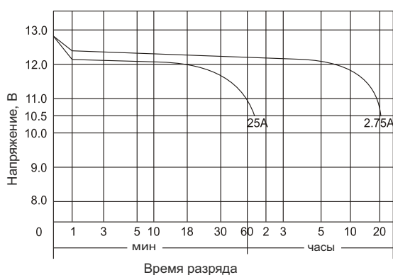
Разрядные характеристики (25°С)
